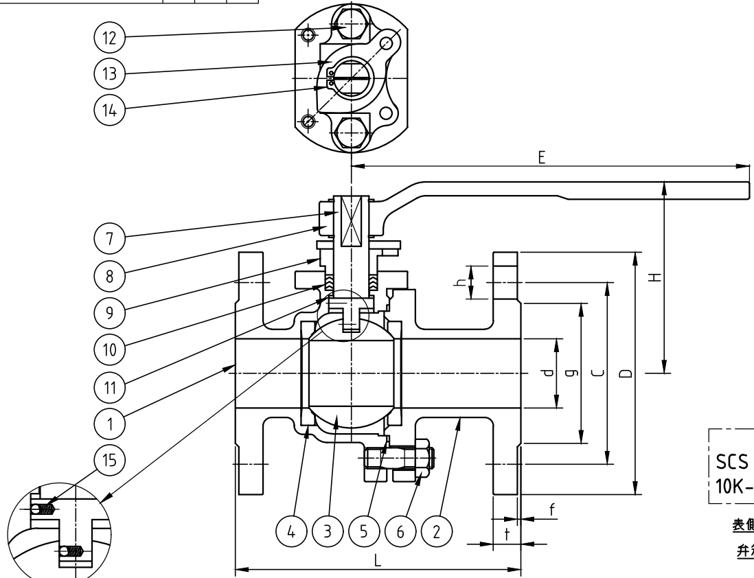
寸法表 単位 (mm)
